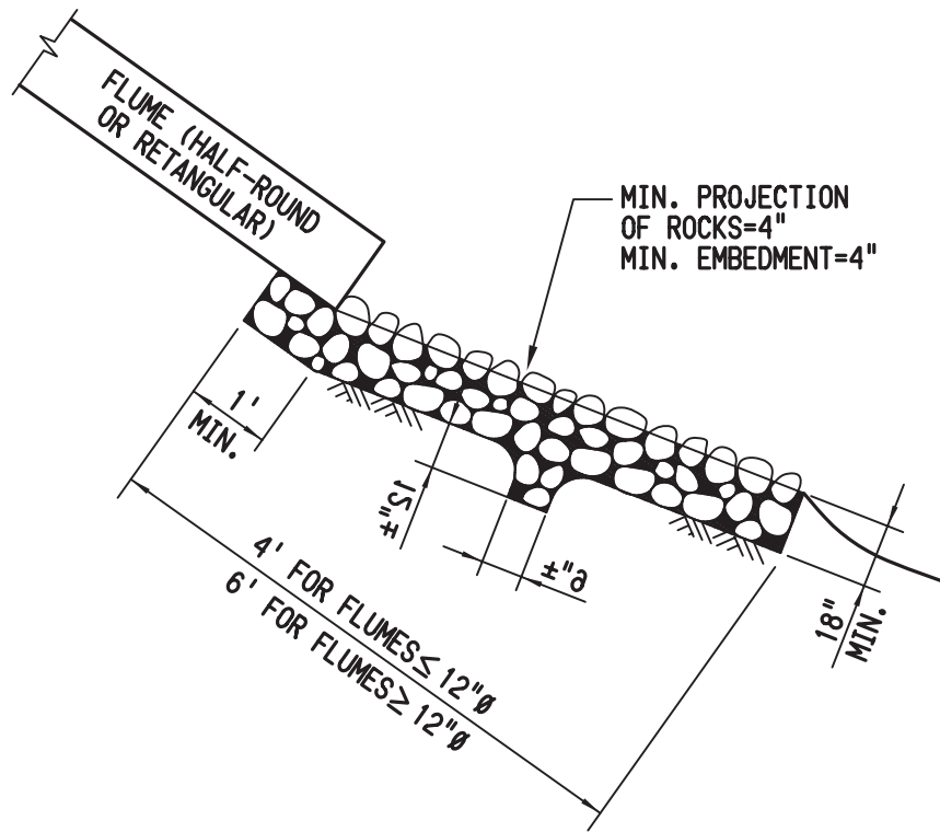
ELEVATION
